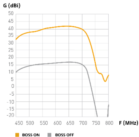
Frekvenssvar
