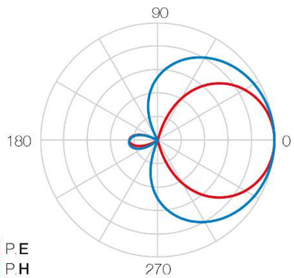
Strahlungsmuster
