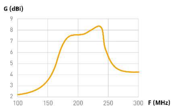
Pasmo przenoszenia
