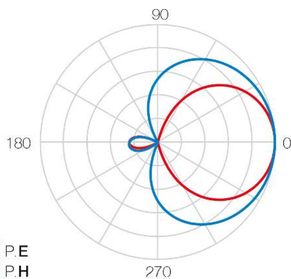
Strålningsmönster
