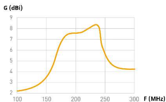
Frekvenssvar
