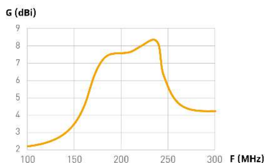
Risposta in frequenza
