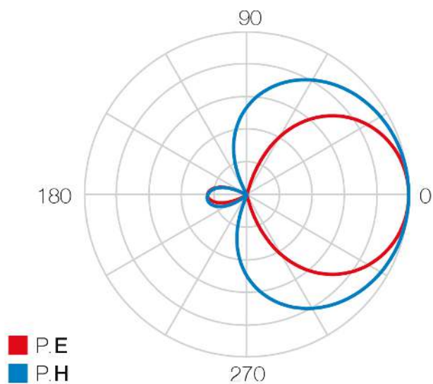
Schema di radiazione
