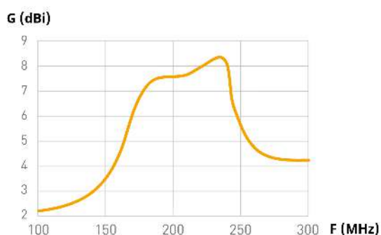
Pasma przenoszenia
