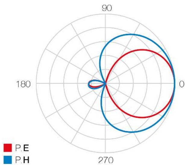
Diagrama de radiação
