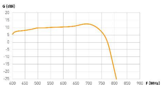
Respuesta en frecuencia
