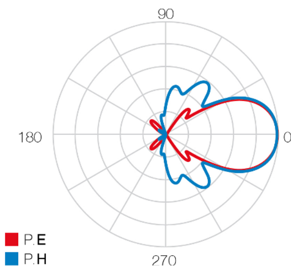
Charakterystyka promieniowania
