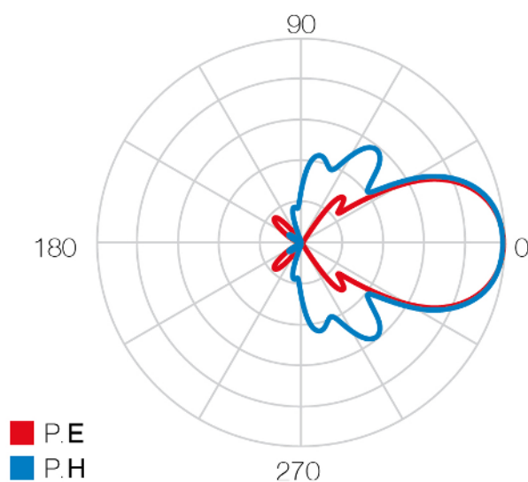
Strålningsmönster
