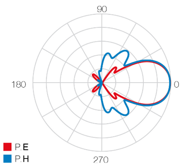
Strålningsmönster
