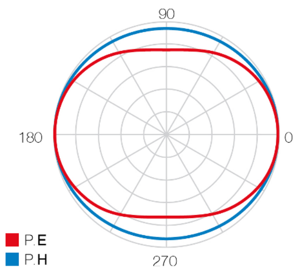
Charakterystyka promieniowania
