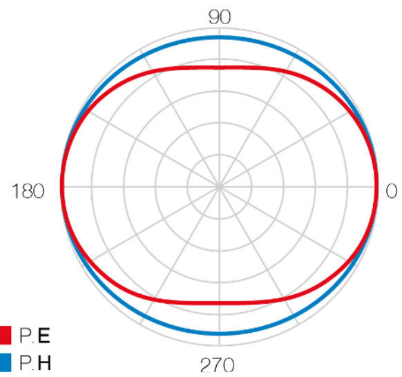
Strahlungsmuster
