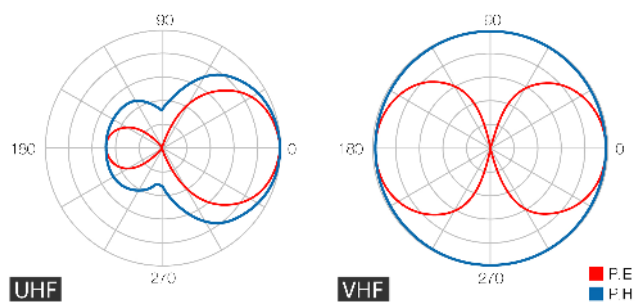
Diagrama de radiación
