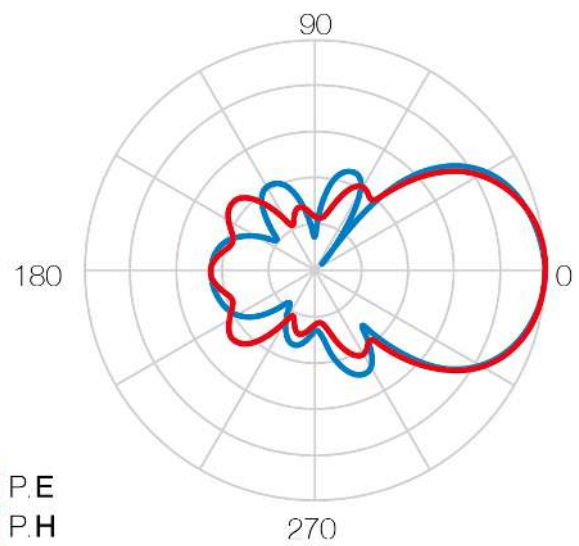
Diagrama de radiación
