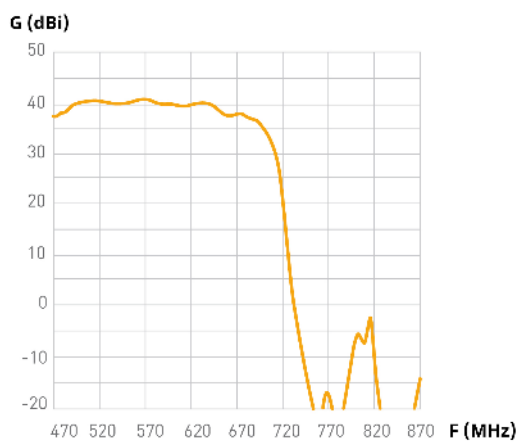
Pasmo przenoszenia
