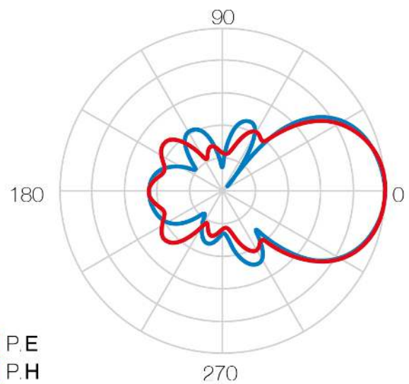
Strålningsmönster
