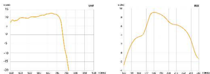
Pasma przenoszenia
