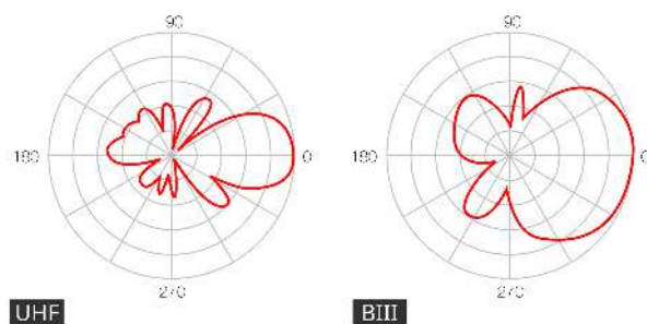
Charakterystyka promieniowania
