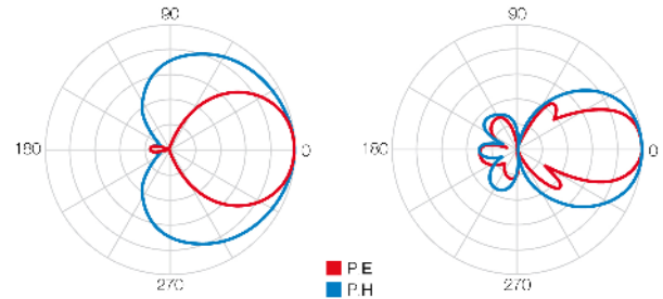
Strahlungsmuster
