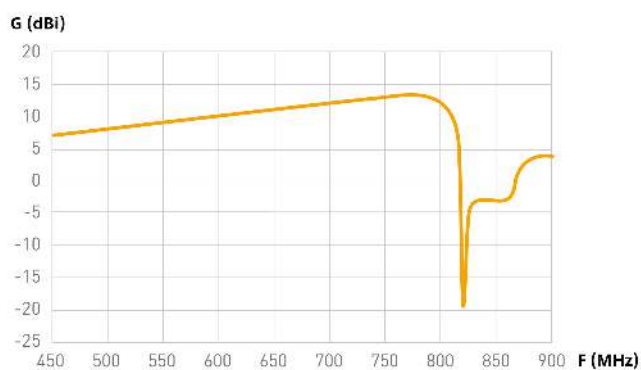
Pasmo przenoszenia
