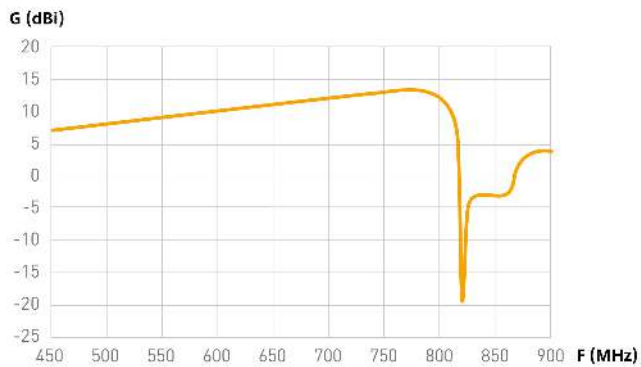
Frekvenssvar
