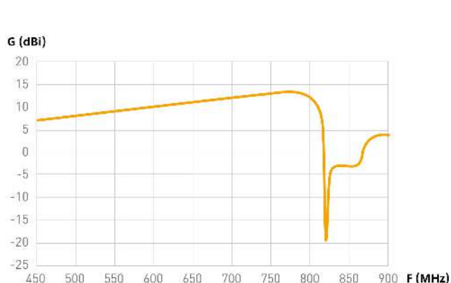
Respuesta en frecuencia
