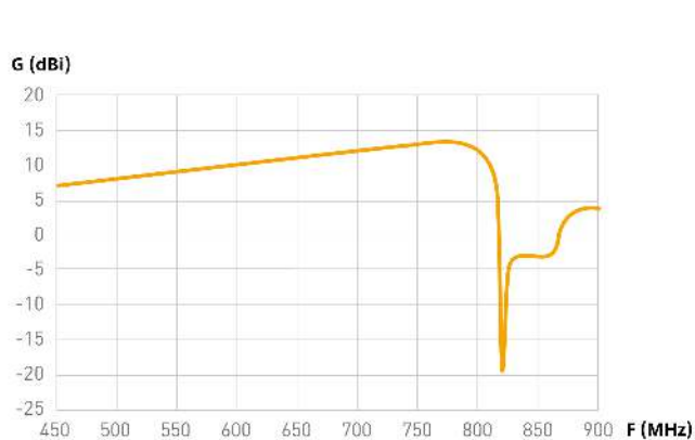
Réponse en fréquence
