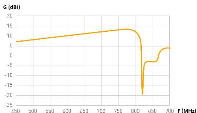
Pasmo przenoszenia
