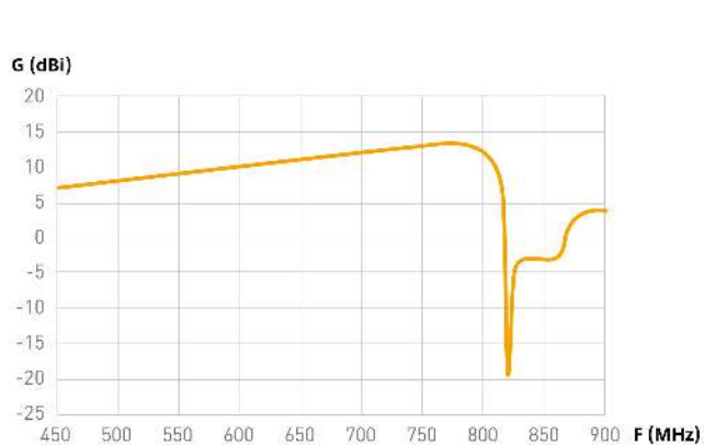
Frekvenssvar
