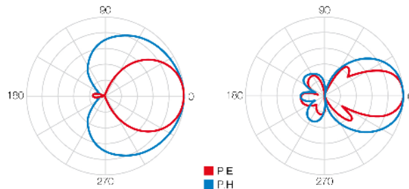
Strålningsmönster
