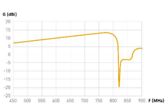
Frekvenssvar
