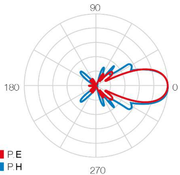
Strålningsmönster
