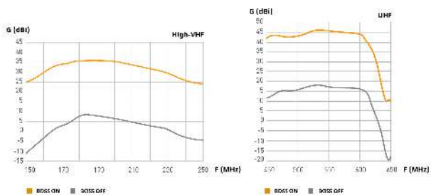
Respuesta en frecuencia
