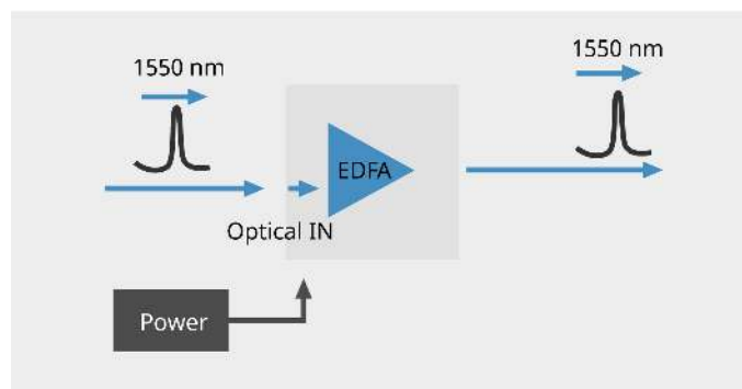
Schemat blokowy
