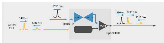
Blockdiagramm
