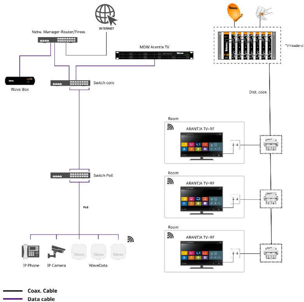
Servicio Arantia TV sobre una red coaxial tradicional + cable Ethernet
