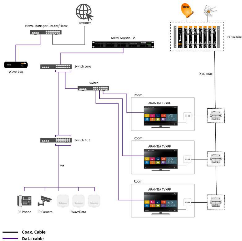
Servicio Arantia TV sobre una red GPON
