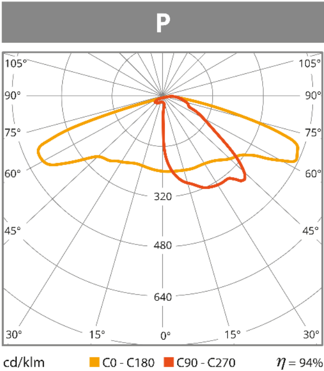
Diffusions lumineuses
