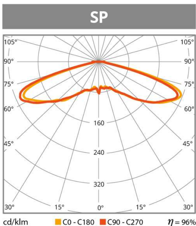
Distribución lumínica
