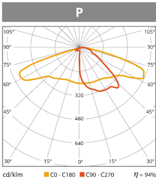
Distribución lumínica
