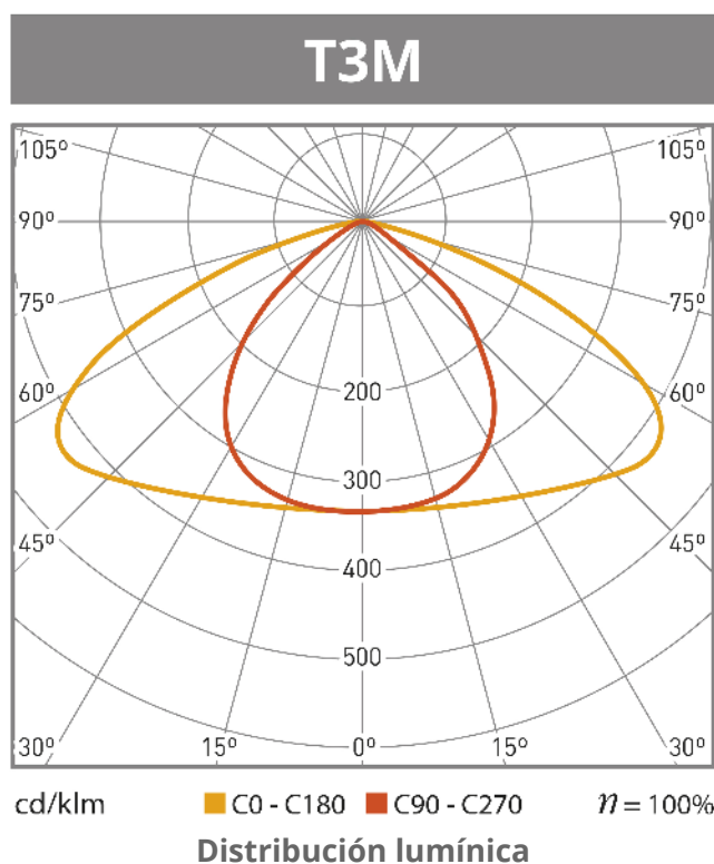
Distribución lumínica
