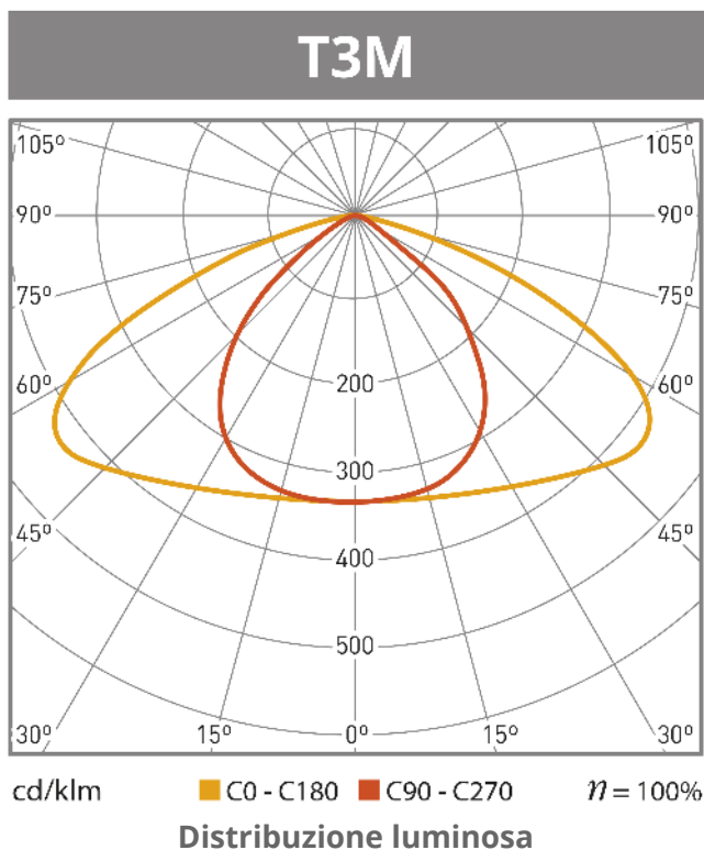
Distribuzione luminosa
