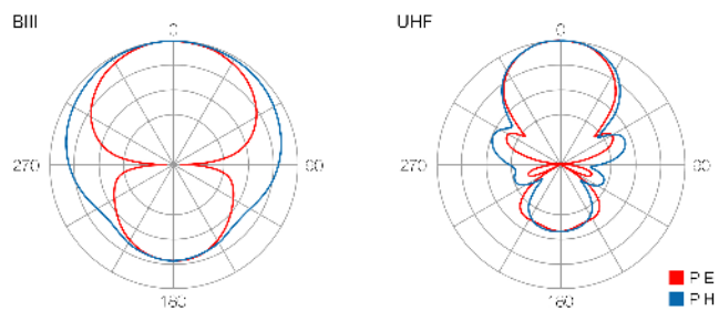
Charakterystyka promieniowania
