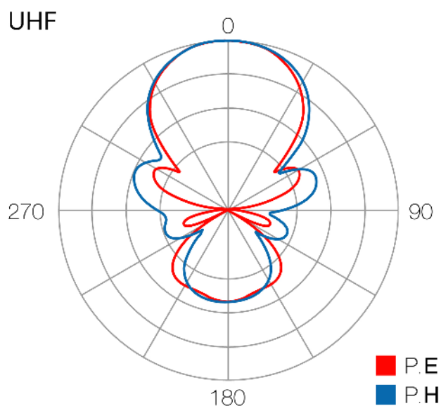
Diagramme de rayonnement
