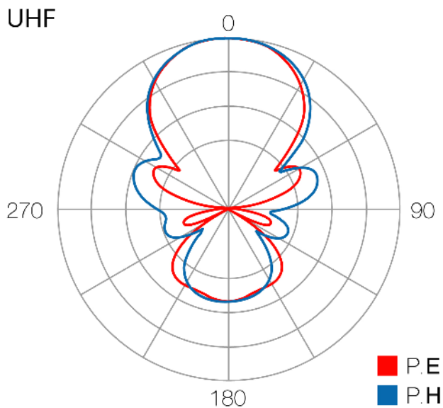
Strålningsmönster
