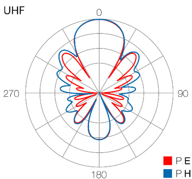
Strahlungsmuster
