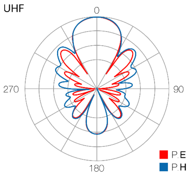
Strålningsmönster
