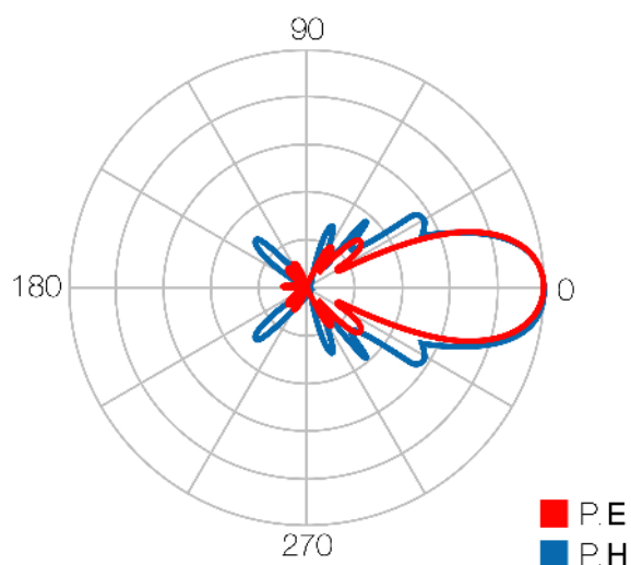
Diagrama de radiación
