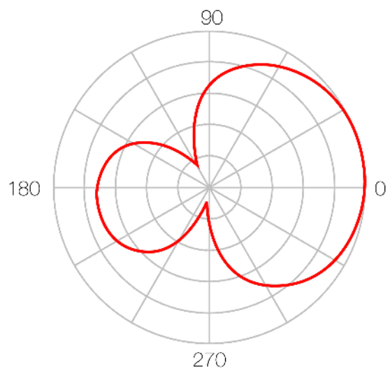
Strahlungsmuster
